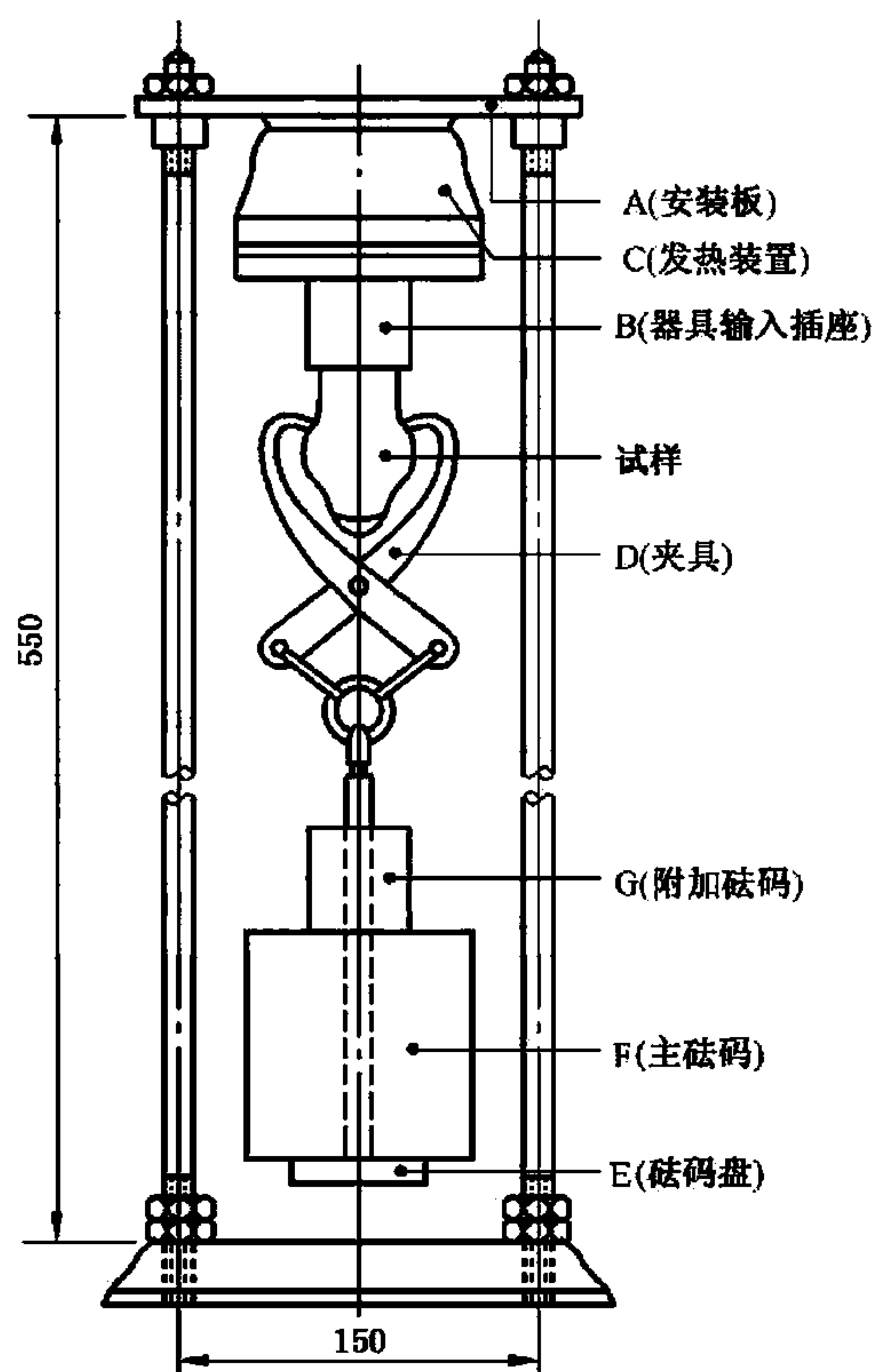
图 11 测试非实心插销用的装置(见 13.4)
