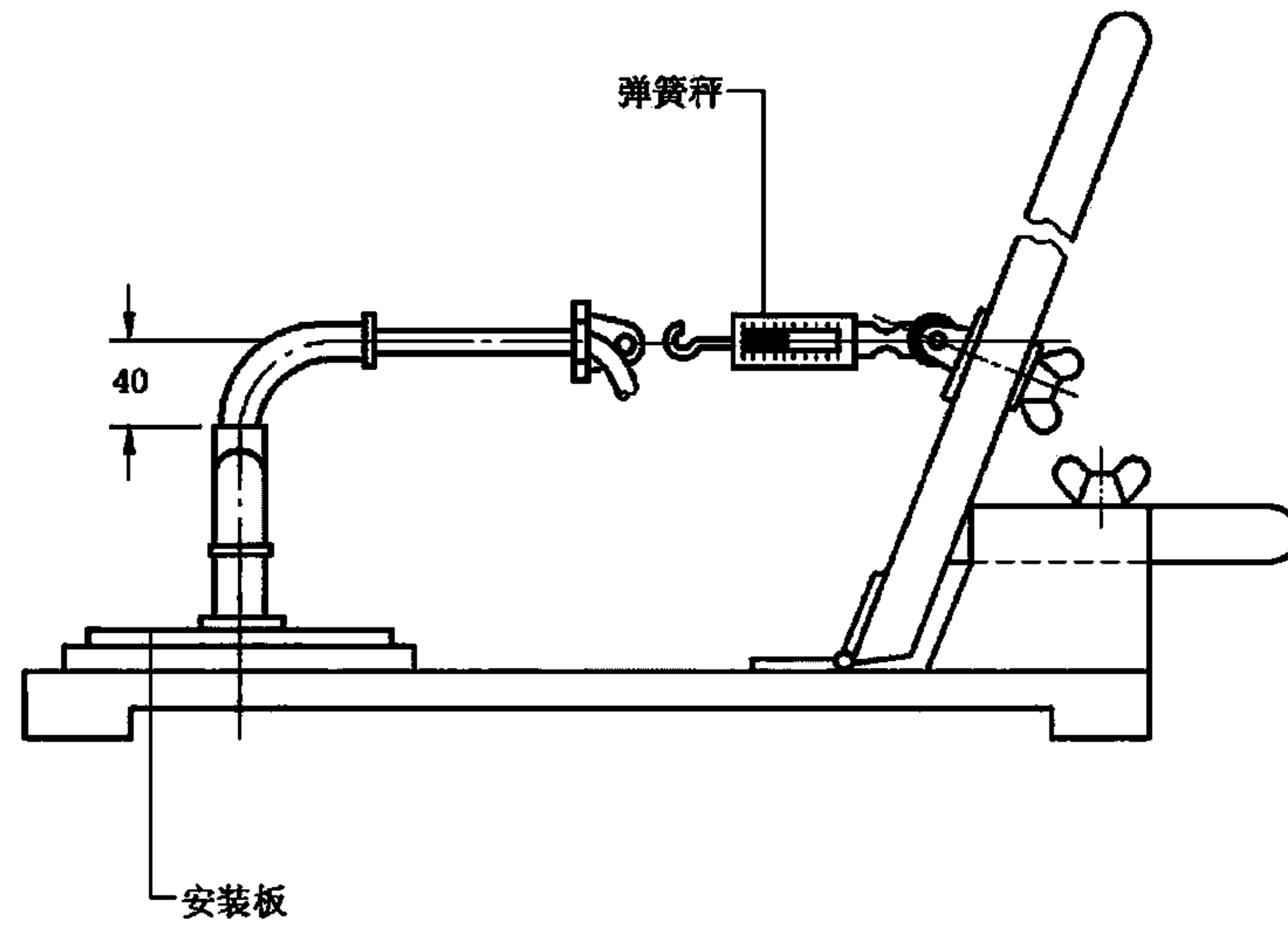
图 19 拉力试验装置(见 23.3)
