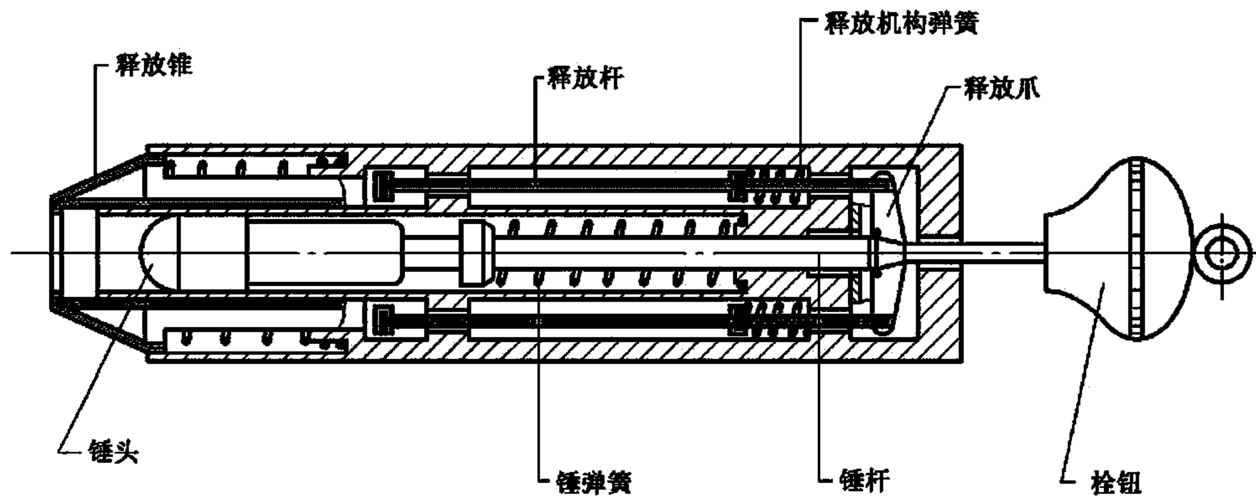
图 21 冲击试验器(见 23.5)
