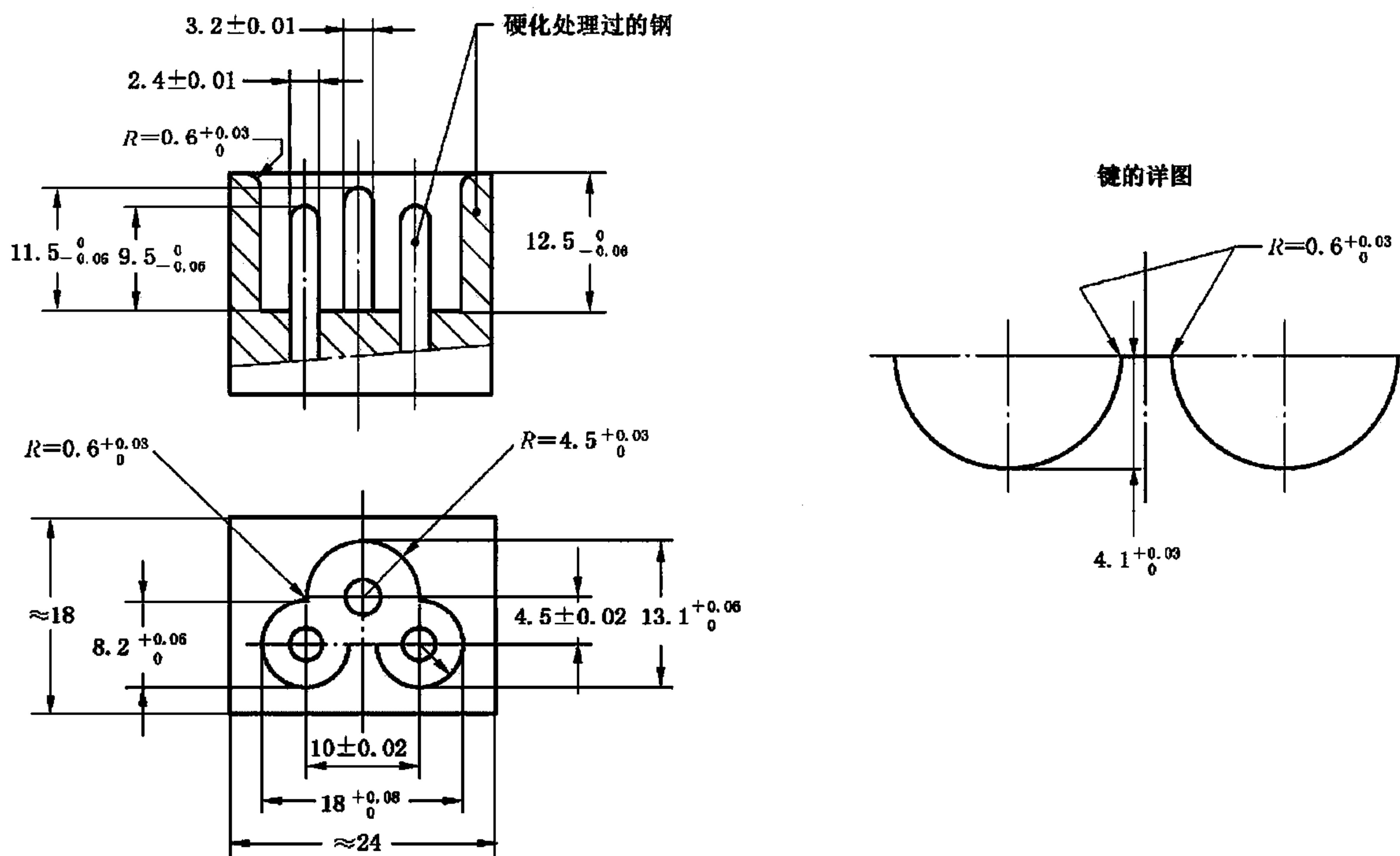
图 2 用于检查连接器是否符合标准活页 C1 的通规(见 9.1)
