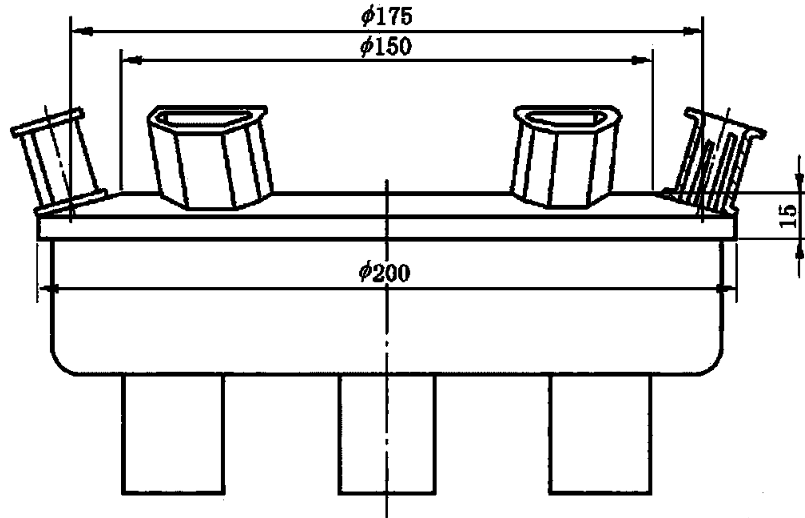
图 13 加热试验用的装置(见 18.2)
