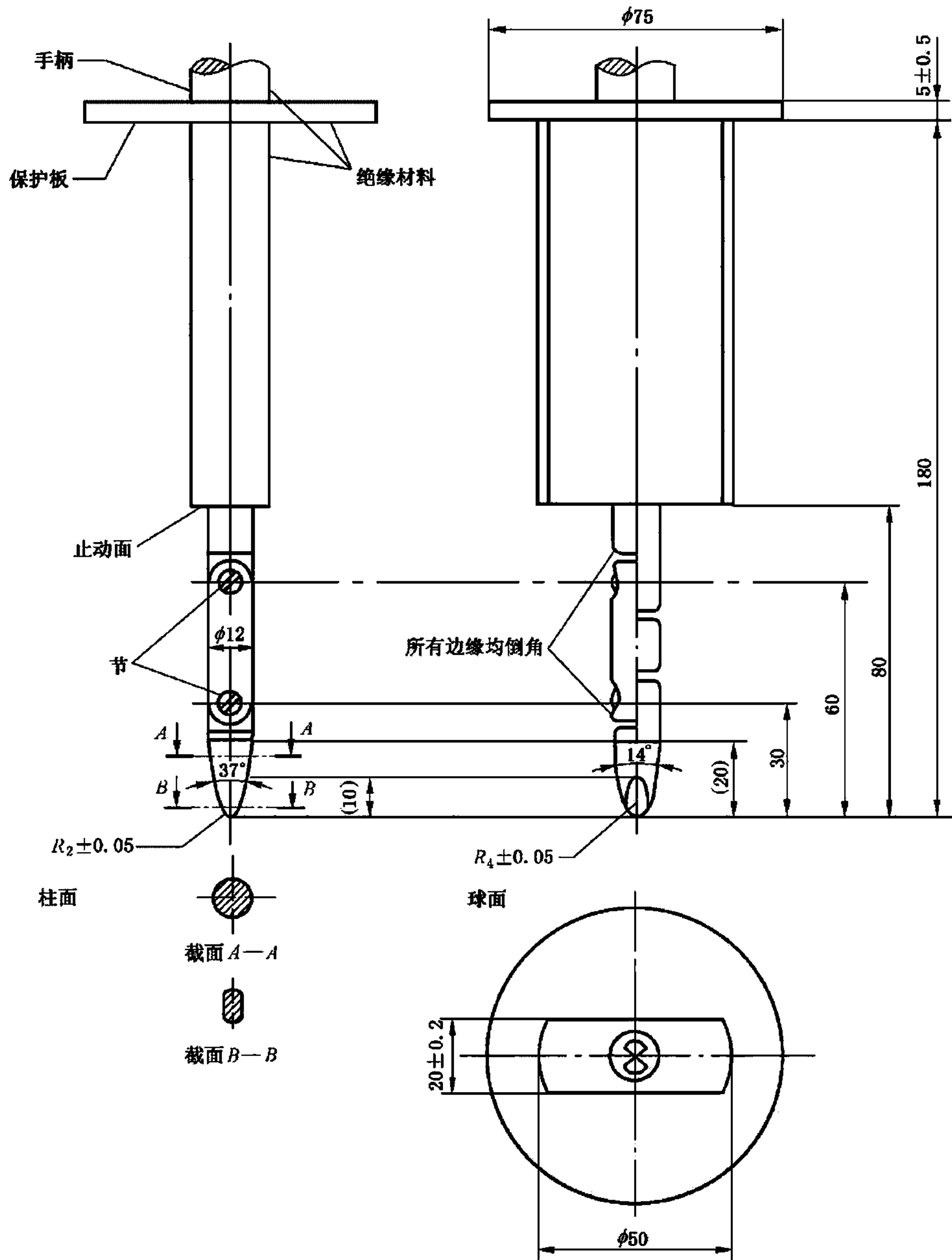
图 10 标准试验指(见 10.1)
