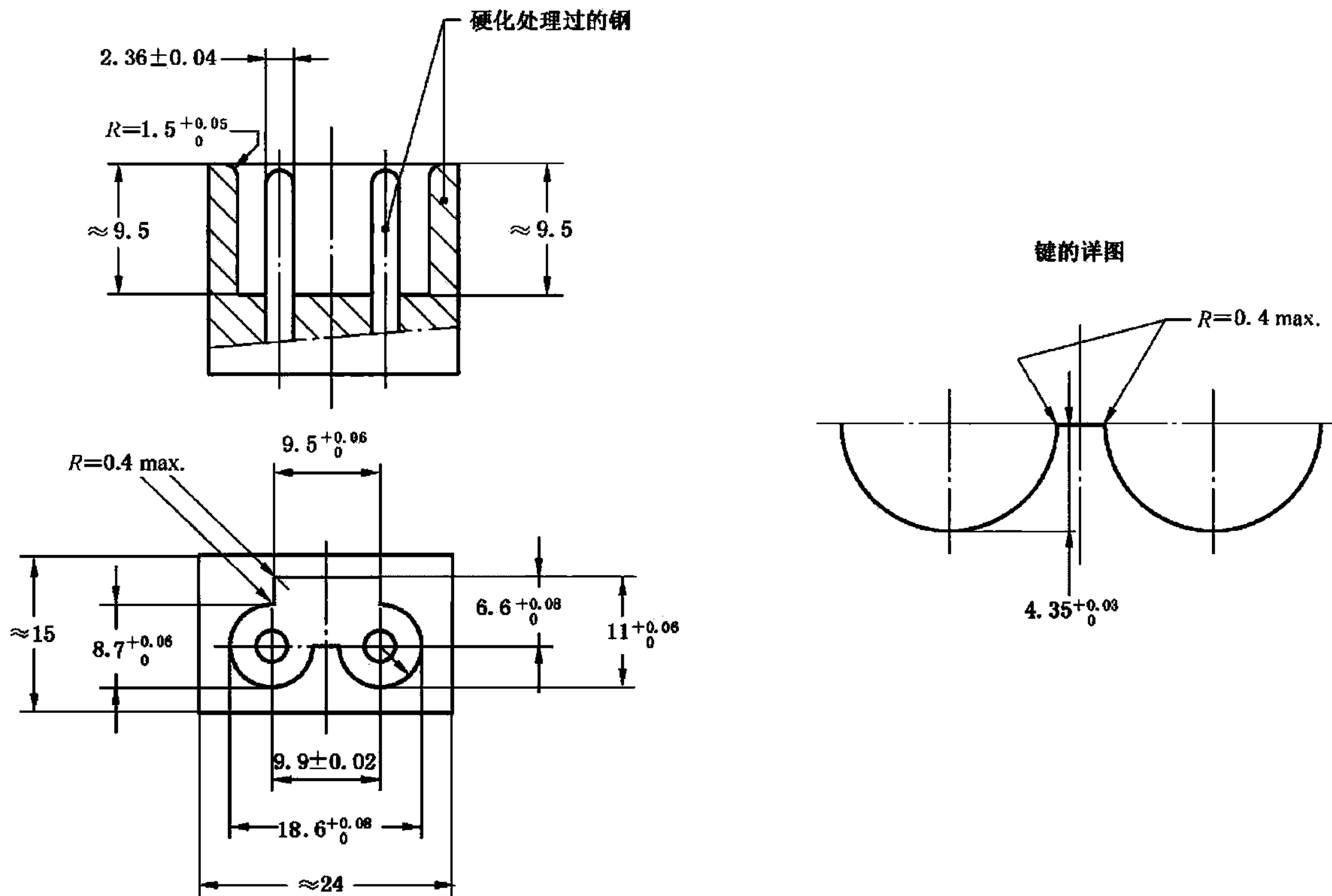
图 6 用于检查连接器是否符合标准活页 C1 的止规(见 9.4)
